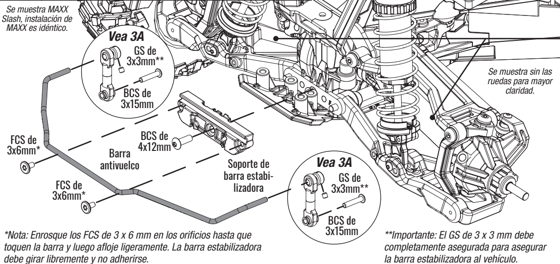
Fig 4 Installation de la barre antirollis arrière
