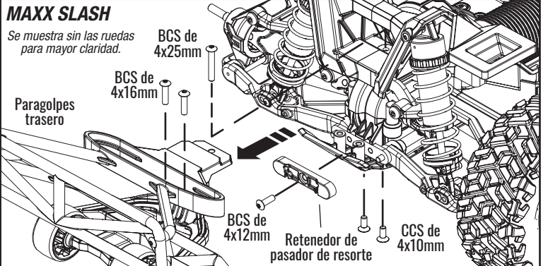
Fig 2 Extracción del retenedor de pasador de resorte trasera
