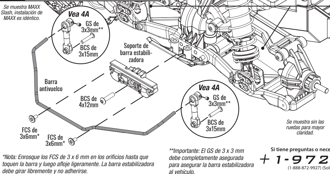
Fig 4 Installation de la barre antirollis arrière
