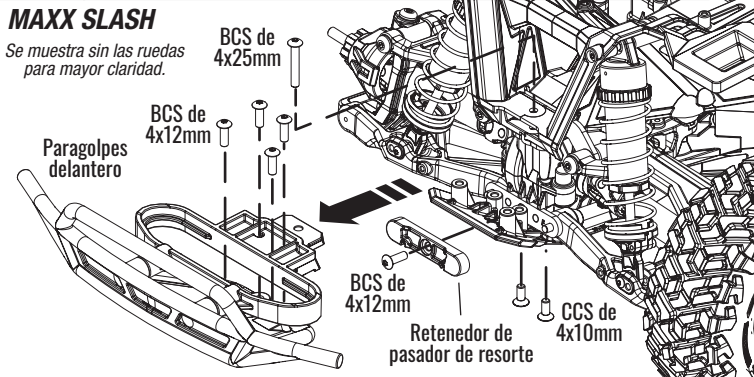
Fig 1 Extracción del retenedor de pasador de resorte delantero
