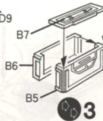
■ CAL.50 탄약상자 CAL.50 AMMO BOX
